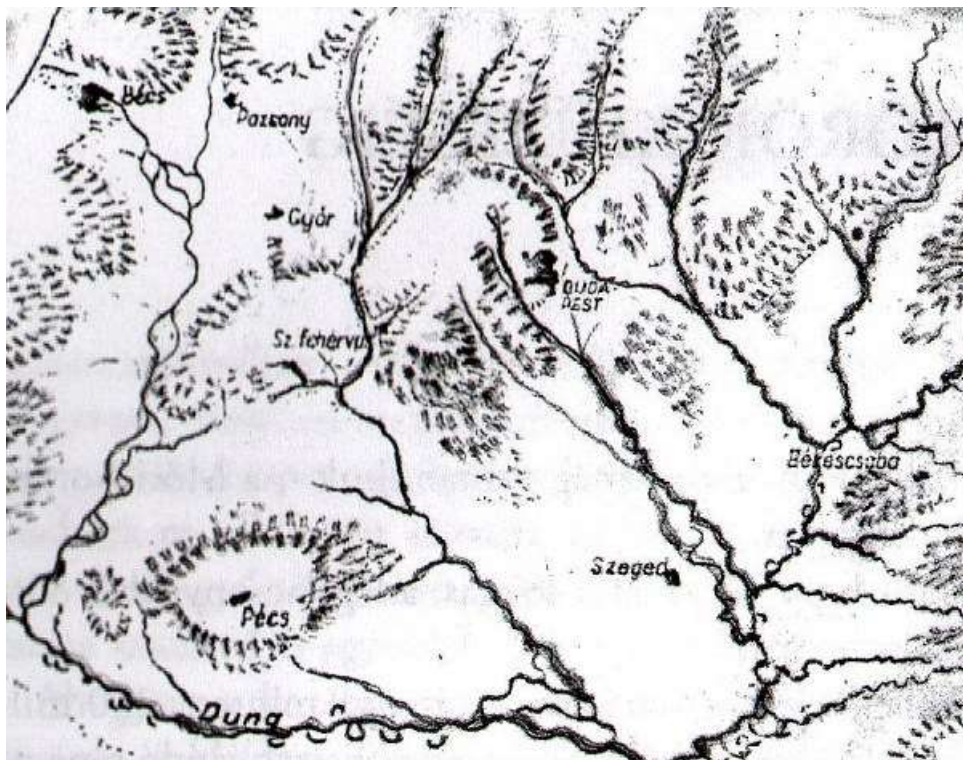
Magyarország ősvízrajza a pleisztocén kor elején
