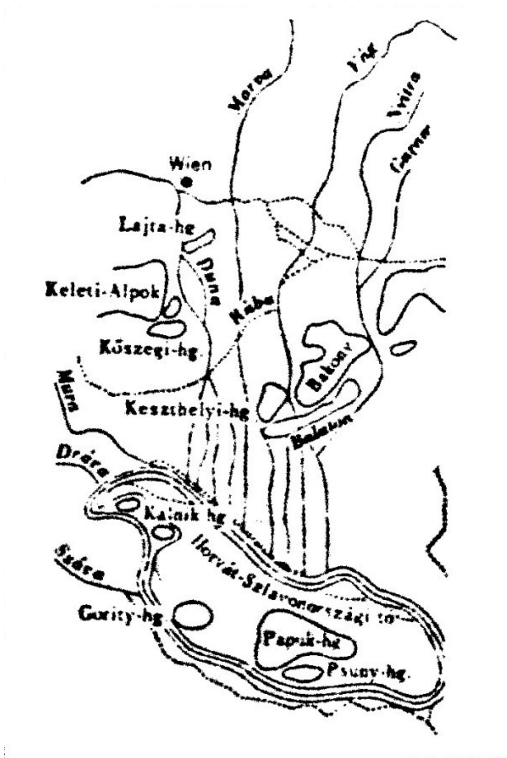
Ferency J. által feltételezett pliocénvégi folyók
